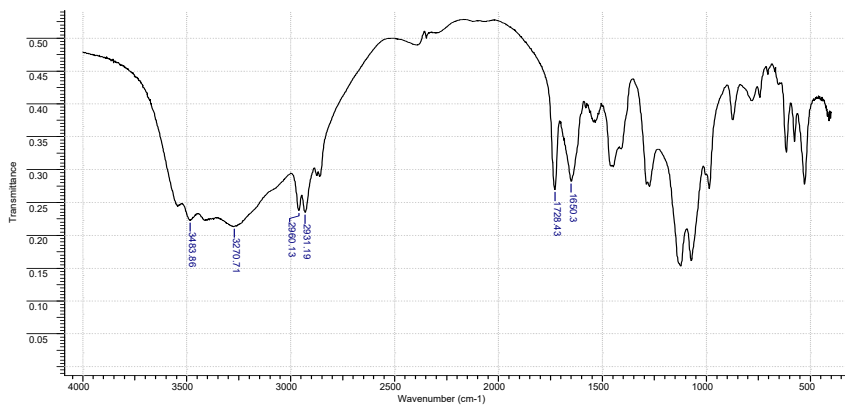
Рис. 1. Пример инфракрасного спектра комплекса пероксидаза-желатин
